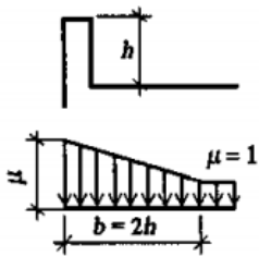
Схема 10. Покриття з парапетами
